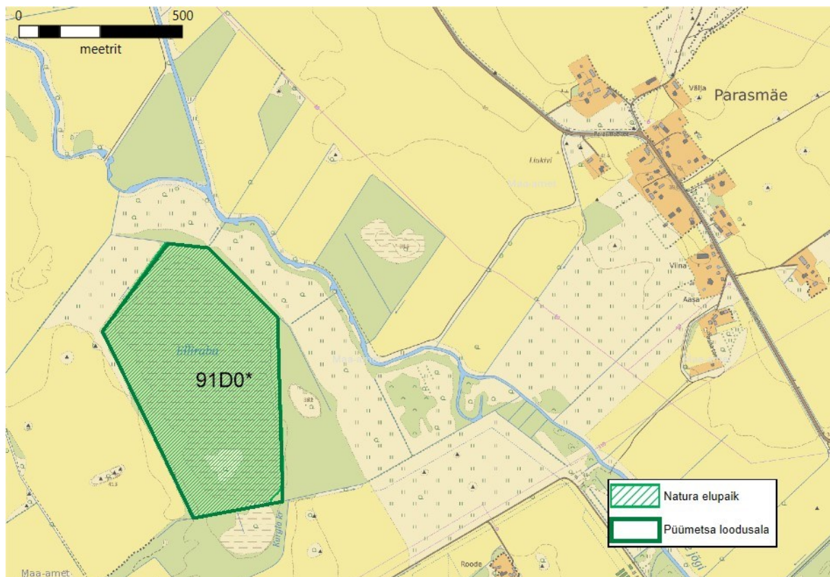
Joonis 1. Püümetsa loodusala ja looduslalal inventeeritud elupaigatüüp siirdesoo- ja rabametsad (91D0*) (piirid: EELIS, august 2023; aluskaart: Eesti Põhikaart, Maa-ameti WMS kaardirakendus, august 2023).
